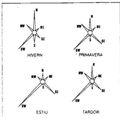
Roses dels Vents d'Olot. Anys 1898-1920. (Elaborades per M. R. a partir de les dades de Quintana.)
