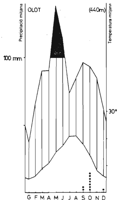
Diagrama climàtic d'Olot. A la part inferior hi ha assenyalats els aiguats anotats pels observadors. (Font: J. M. Panareda. Geografia física dels PPCC).
