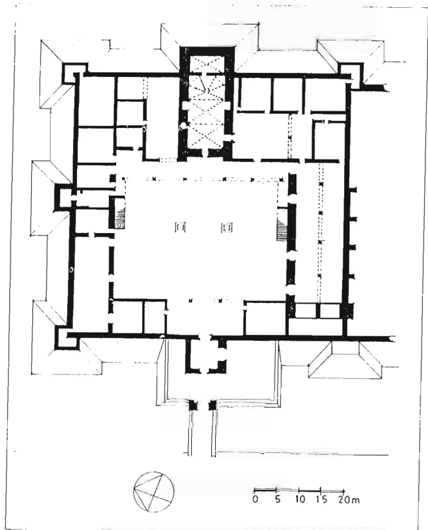
Planta del Palau dels Reis de Mallorca a Perpinyà
