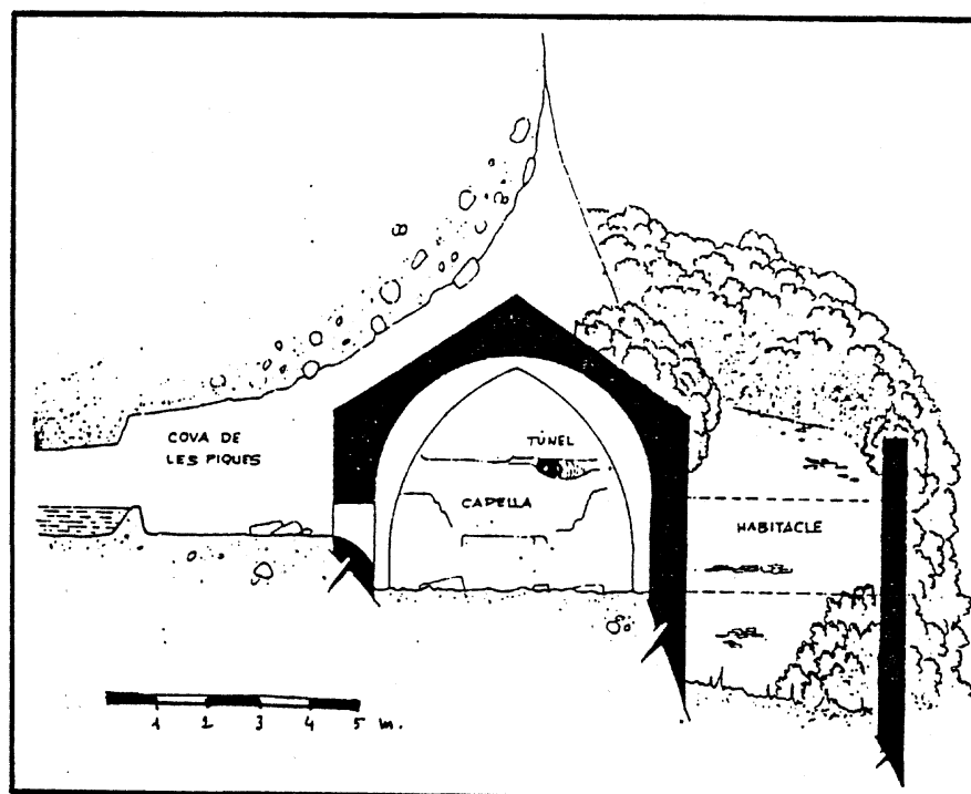
Secció de la cova de Santa Agnès. E: 1/100 - Dibuix d'Antoni Ferrando i Roig
