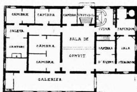
FIG. 3 — PLANTA DEL PIS PRINCIPAL DE LLONGARRIU
