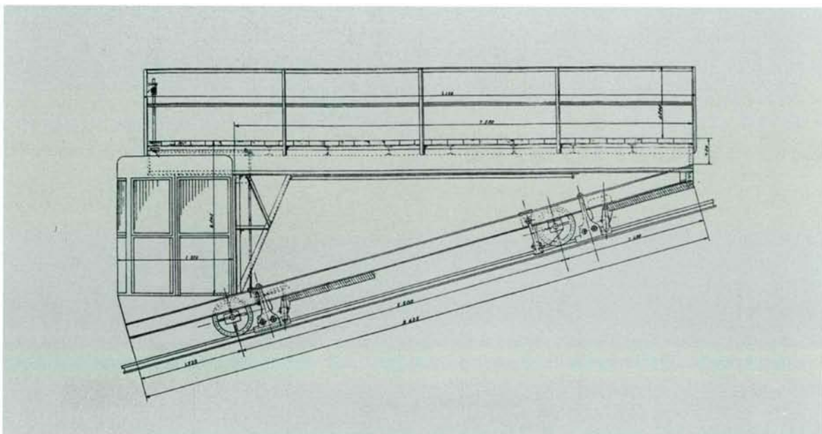
Vista lateral d'un cotxe del funicular comú Sanatori-Hotel, segons el projecte de Locomoción y Transportes (ADB).
