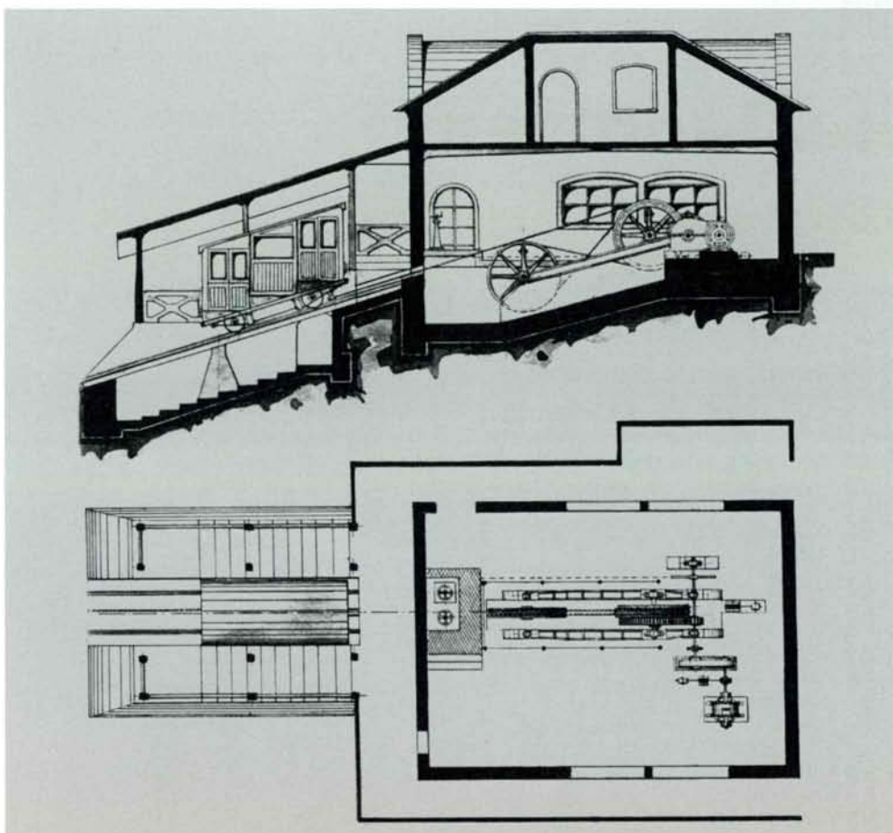
Planta i alçat de l'estació superior del funicular per al sanatori proposat per J. Rodríguez Roda-Ceretti & Tánfani (ADB).
