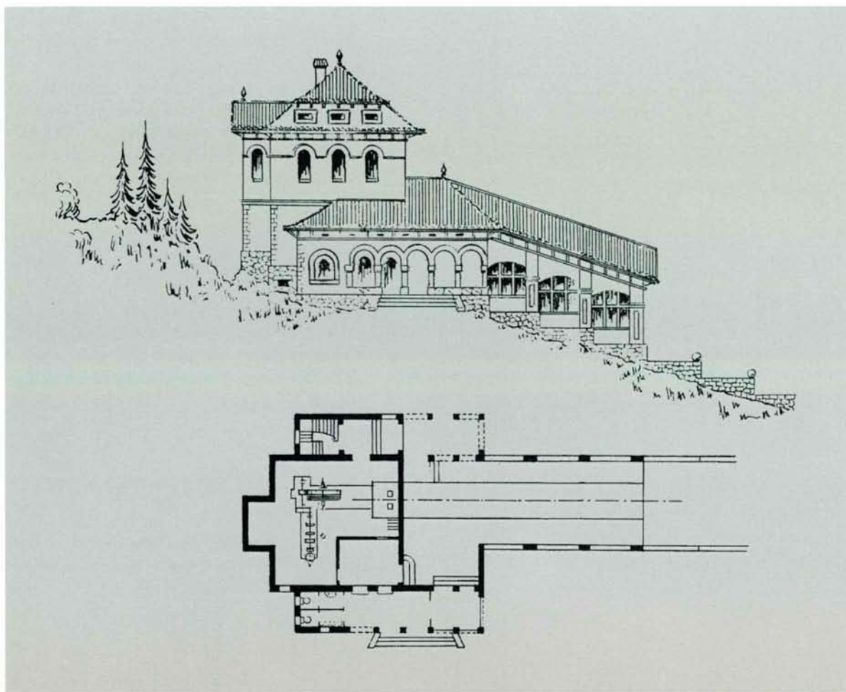
Planta i alçat de les estacions superiors dels funiculars projectats per E. Remy (ADB).
