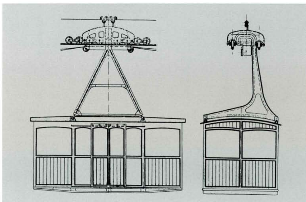
A dalt, vista lateral d'una locomotora a cremallera de la línia Tordera-Sanatori, segons el projecte presentat per Ribera & Cia. A baix, cabina de 40 places del projecte de telefèric proposat per J. Rodríguez Roda per a la línia Gualba-Hotel (Arxiu Diputació de Barcelona).
