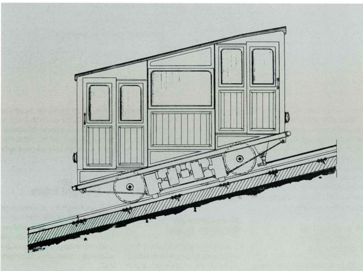
Dibuix en alçat d'un dels cotxes del projecte J. Rodríguez Roda-Ceretti & Tánfani (ADB).
