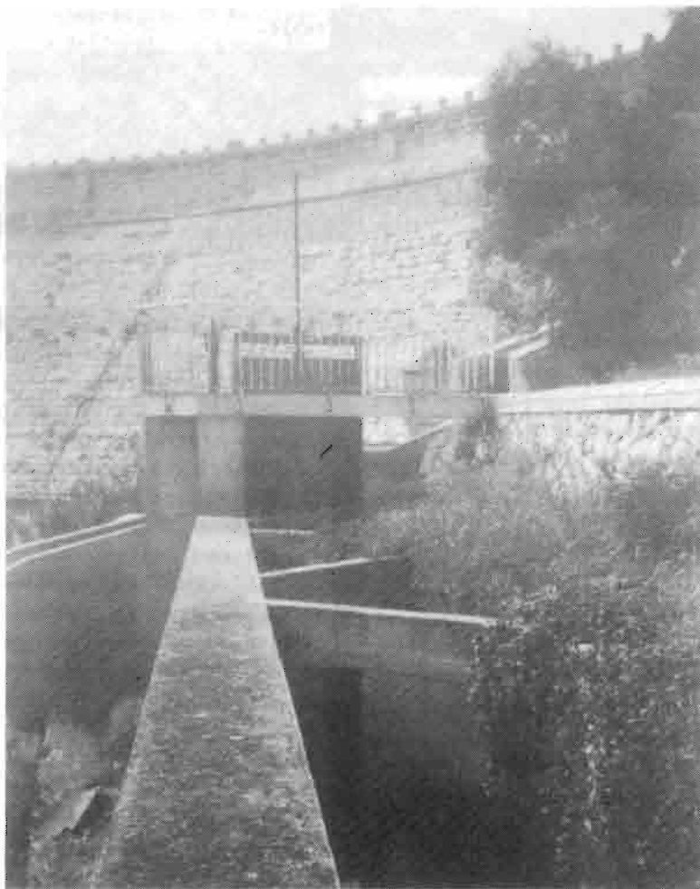
Un dels canals de sortida del Pantà. Al fons la presa. (Foto: J. Sivill)
