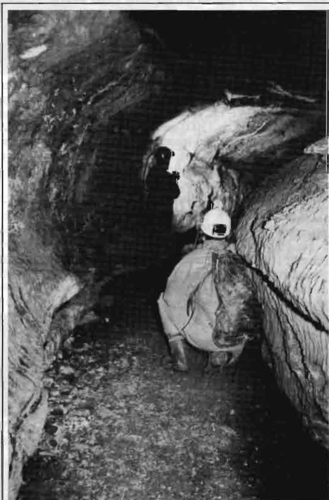
Mari-ko Leizea. Conduite subterrani d'un riu fossilitzat. Foto: J.J.Melgarejo
