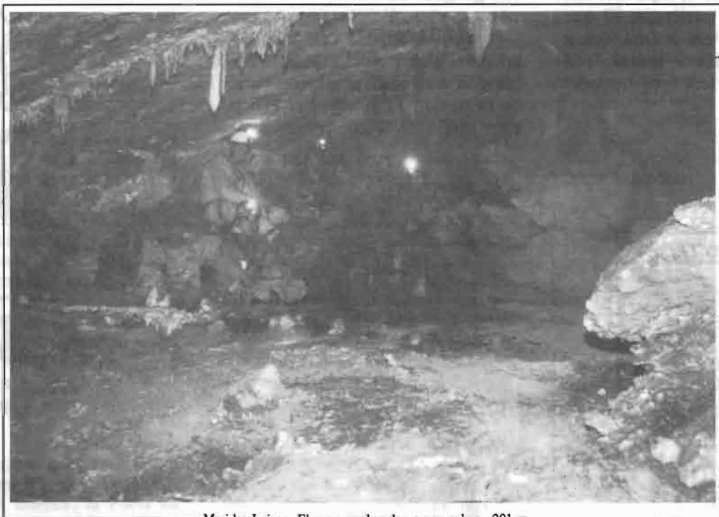
Mari-ko Leizea. El grup explorador a una sala a -201 m. Foto: J.J.Melgarejo
