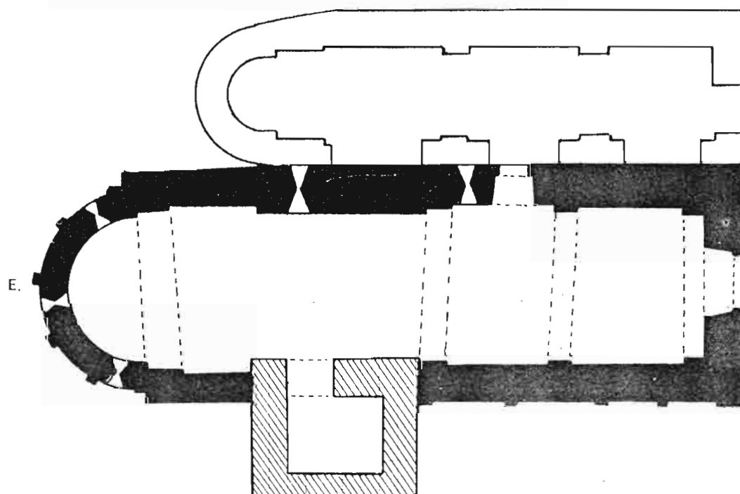
Planta de l'església de Sant Climent de COLL DE NARGÓ
