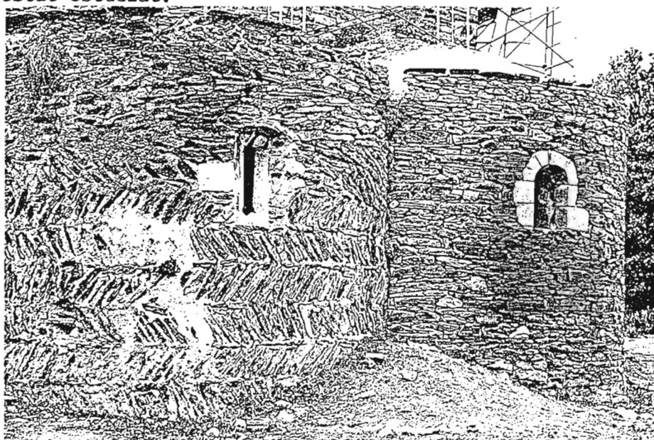
Santa Coloma de Fitor. Capçalera exterior de l'església, on és perfectament visible l'opus spicatum (foto: A. Borbonet)
