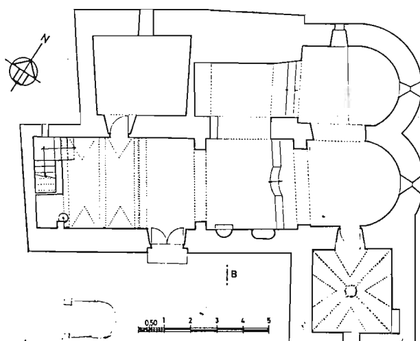
Santa Coloma de Fitor. Planta del conjunt de l'església, a escala 1:200 (planta: Ll. Bayona-Servei de Conservació de Monuments de la Diputació de Girona)
