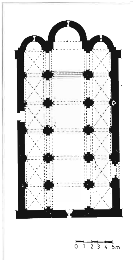
Planta de l'església de Santa Maria d'Ovarra, extret de La España Románica. Aragón .
