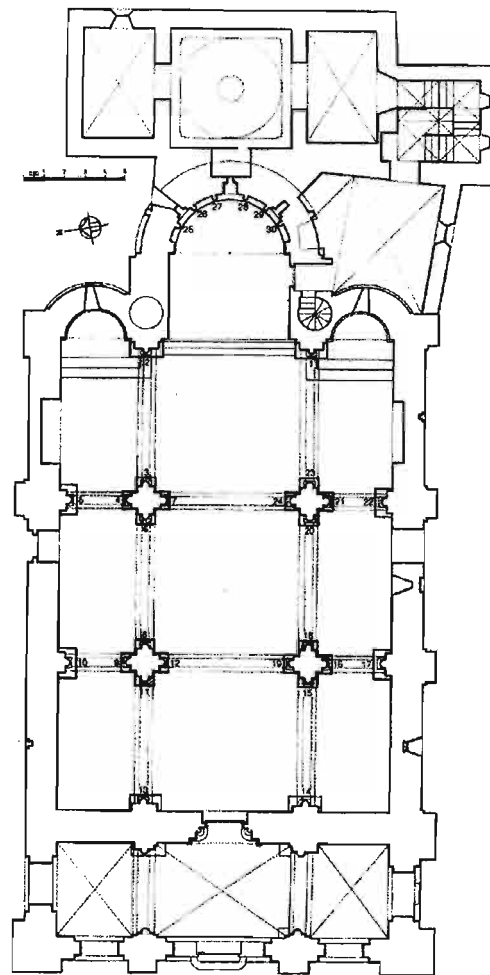
Planta de l'església del monestir de Santa Maria de Gerri de la Sal, Catalunya Romànica
