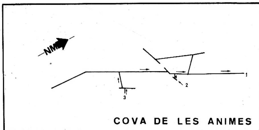
Fig. 2.— Esquema de la anemocirculación que afecta a la Cova de les Animes. 1 y 2, bocas A y B respectivamente de la Cova de les Animes I, y 3, boca de la Cova de les Animes II. Entrada de aire en 2 y 3 en dirección a 1.
