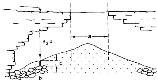
Fig. 4. — Disposición de los pocillos de degoteo en la masa de nevé. a) zona carente de pocillos; b) materiales clásticos englobados en la masa de nevé.
