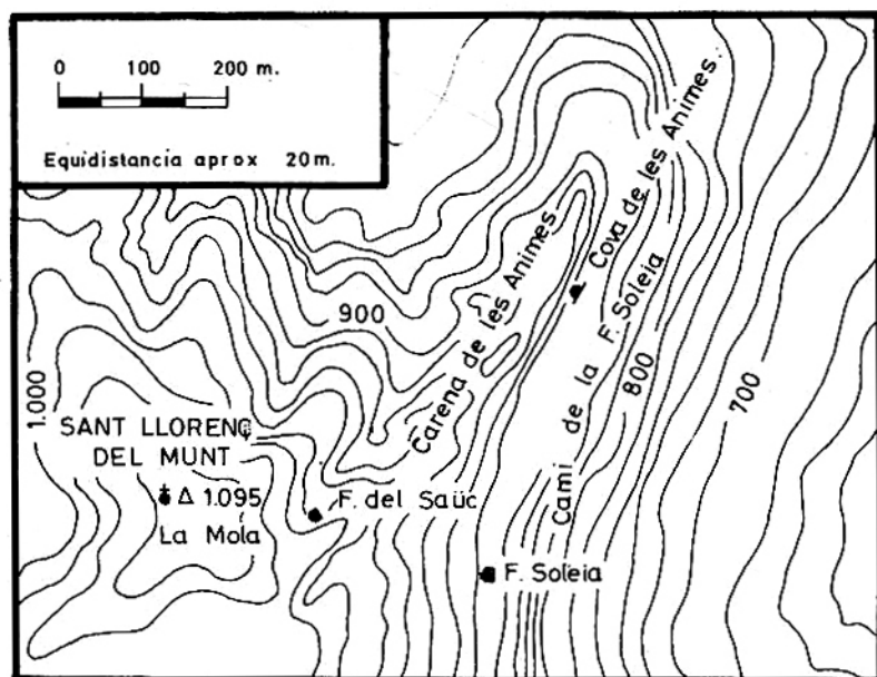
Fig. 1.— Situación geográfica de la Cova de les Ànimes.
