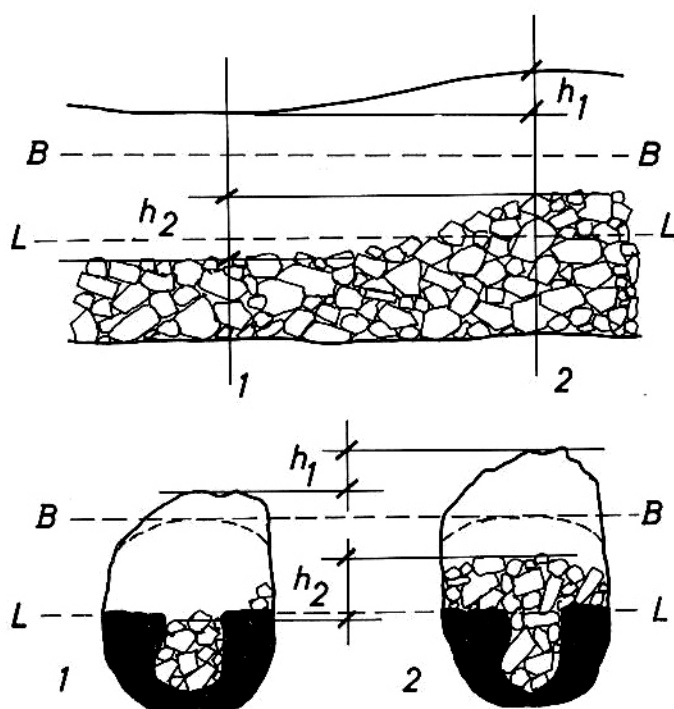
Fig. 5.—Relaciones entre la geometría de la bóveda y los productos clásticos. Ver explicación en el texto.
