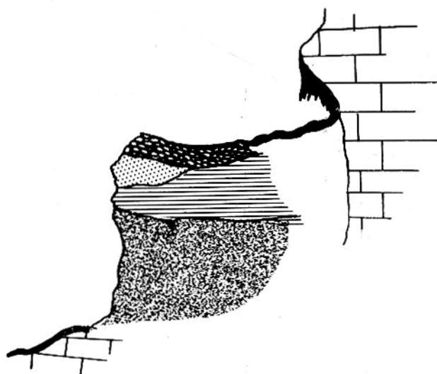
Fig. 4. — Corte estratigráfico. Punto X.
