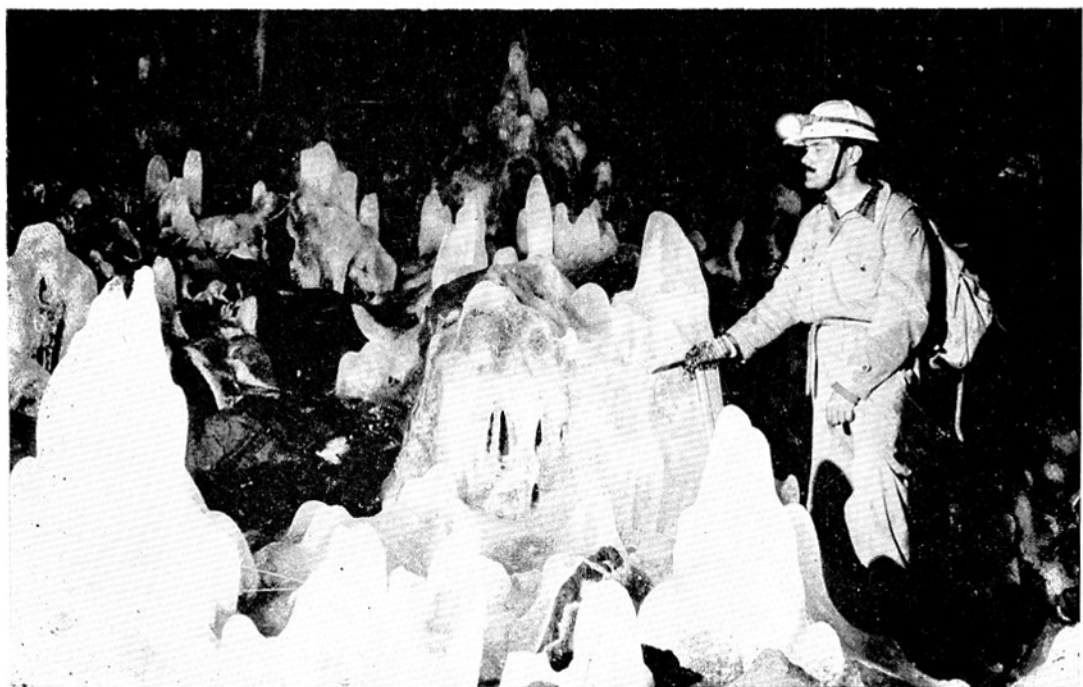
Formaciones de nieve desarrolladas en el fondo de los jameos C y D. (Foto 1). Bosque de estalagmitas de hielo, situado entre las secciones 4 y 5 (ver planta, fig. 1). (Foto 3).
