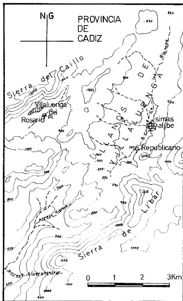
Fig. 1.— Situación de las cavidades.
