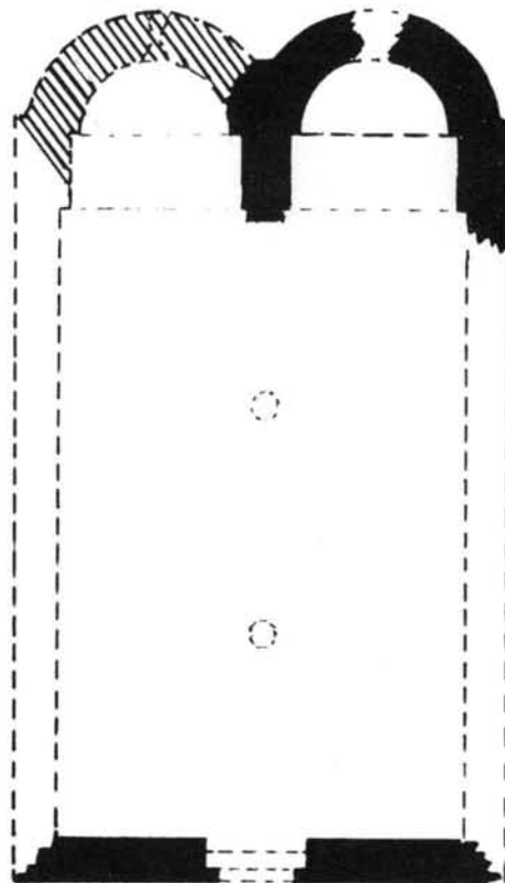
Sant Bartomeu de Baiasca, planol esquemàtic. (Dibuix de Joan Rals.)
