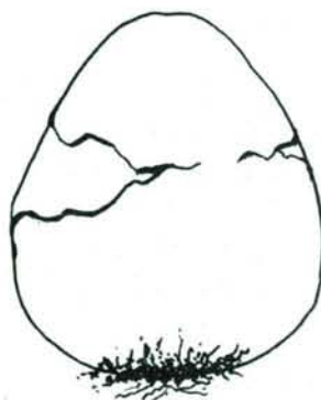
En l' Amanita phalloides , la part més estreta de l'ou, apunta cap amunt.
