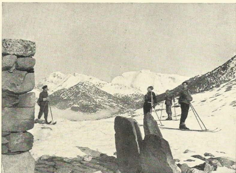
Tucs de Montoliu i Mauborne, des de l'Orri dels Gavatzos
