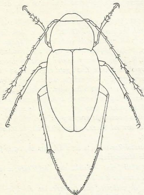
Fig. 1. Speophilus Kiesenwetteri s. str. Dieck. mascle (x 20)
